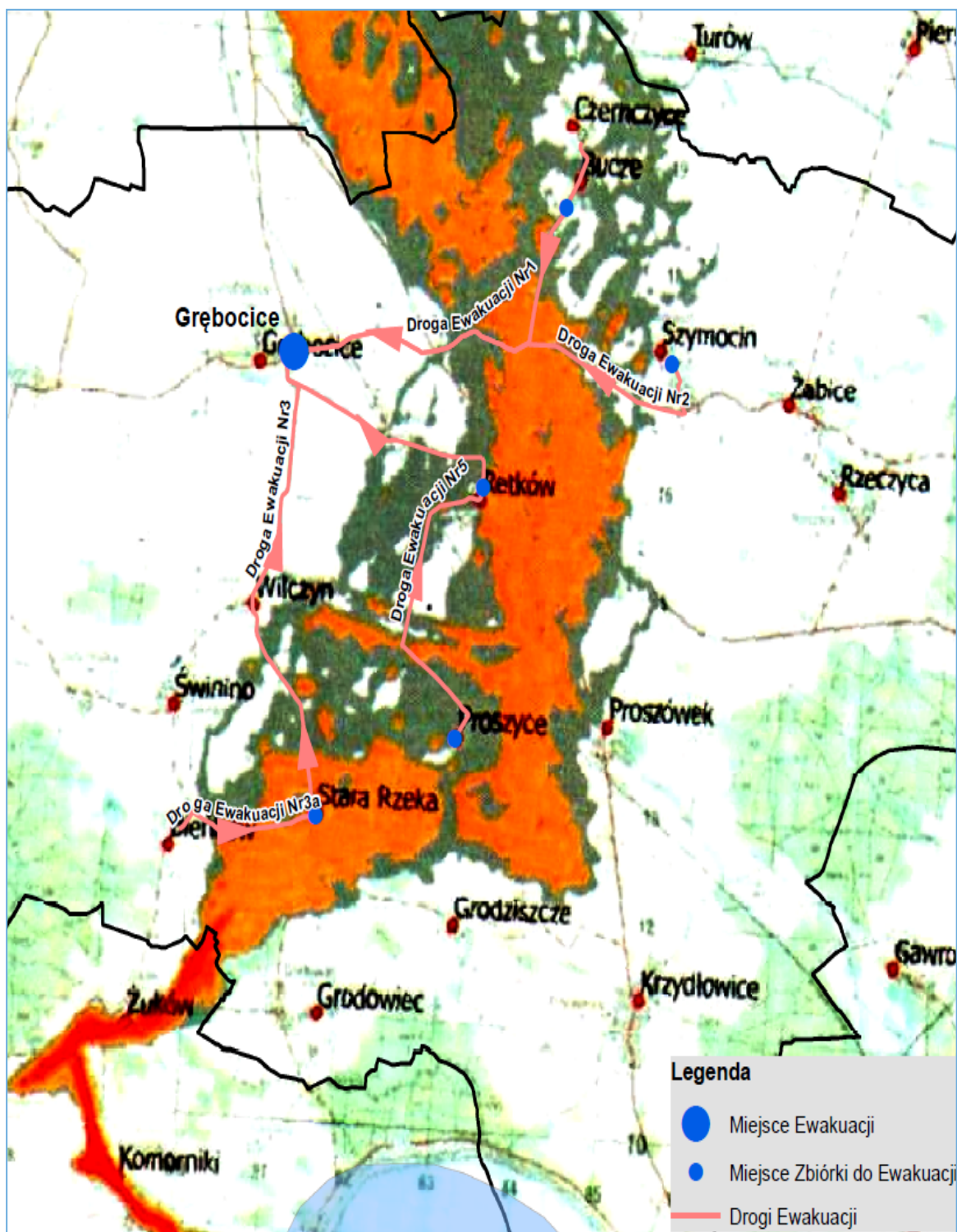
Rysunek 1. 4. Scenariusz 4 – Awaria zapory zachodniej OUOW Żelazny Most
