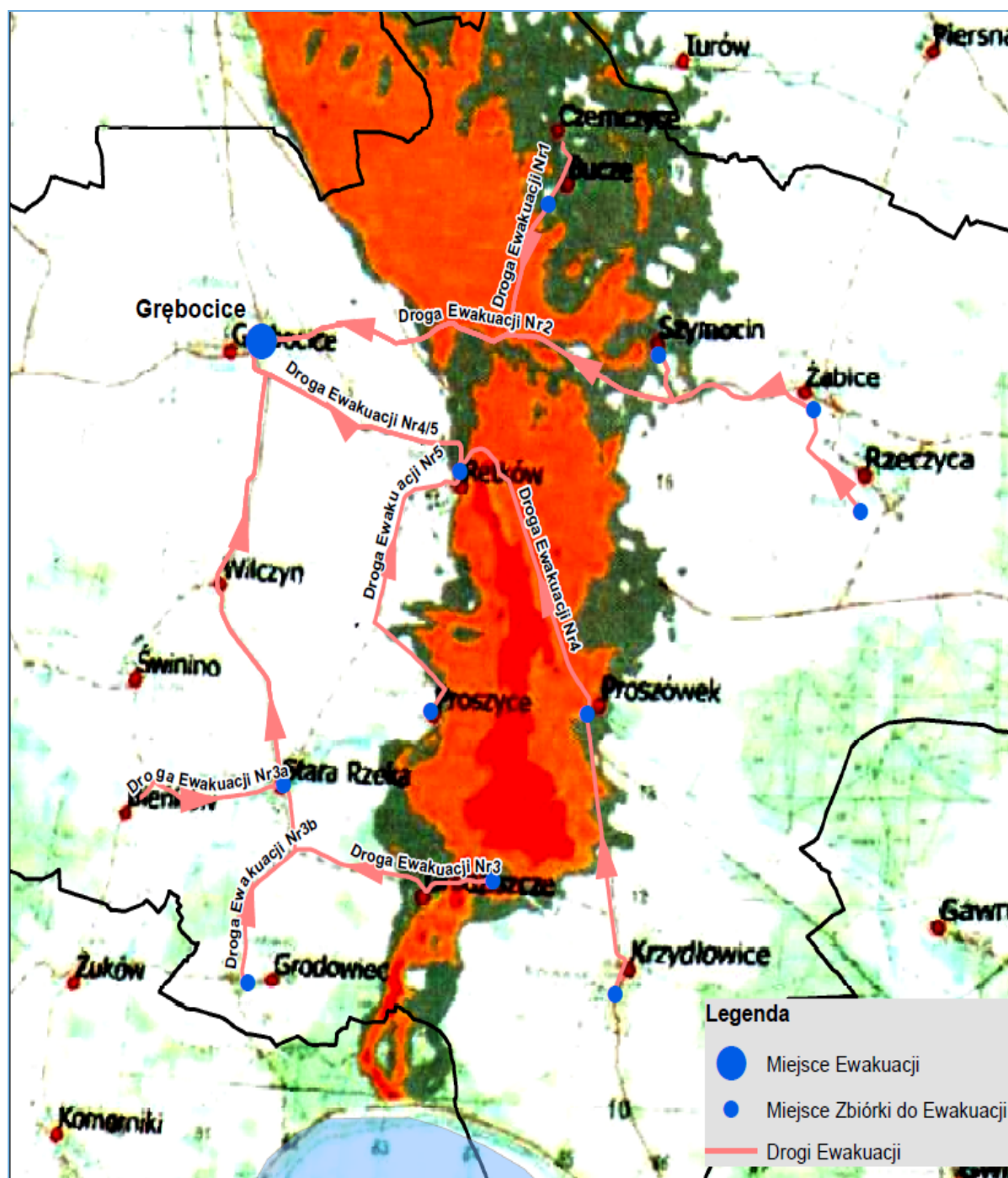
Rysunek 1. 1. Scenariusz 1 – Awaria zapory północnej OUOW Żelazny Most
