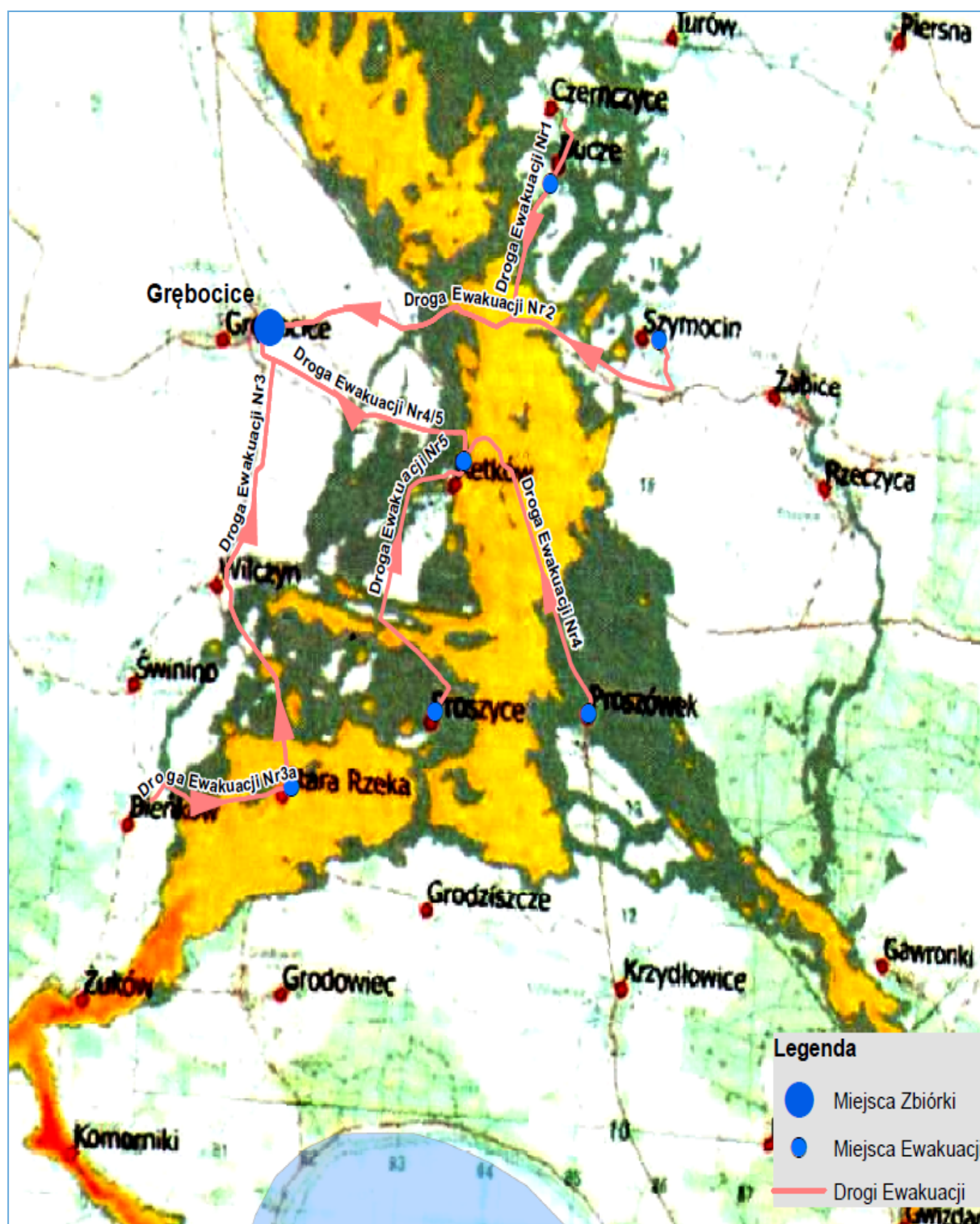
Rysunek 1. 2. Scenariusz 2 – Awaria zapory południowej OUOW Żelazny Most
