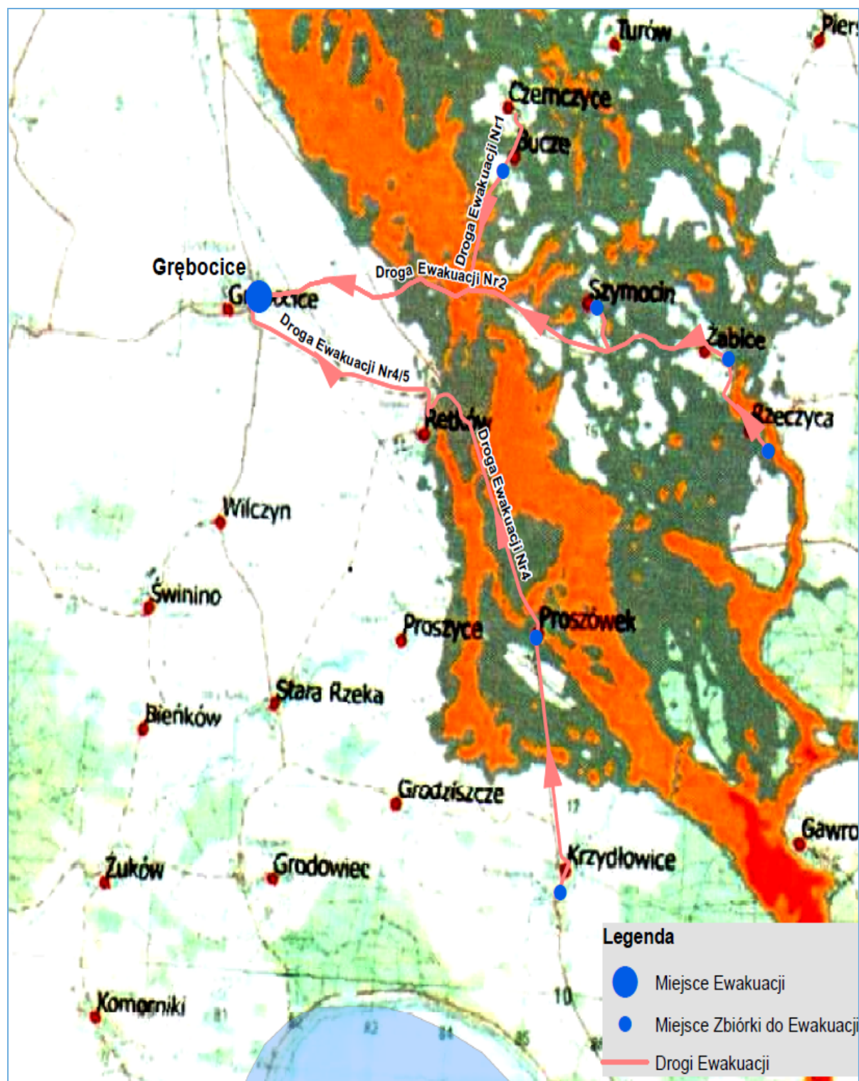
Rysunek 1. 3. Scenariusz 3 – Awaria zapory wschodniej OUOW Żelazny Most
